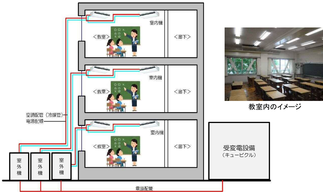
小中学校エアコン設置 イメージ図
