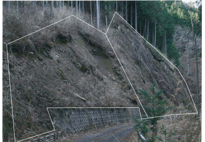
林道樫ノ木峠線(法面吹付工等)
