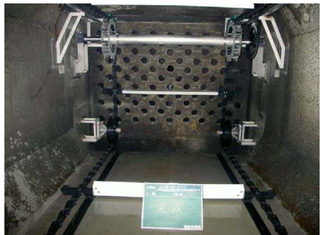
設備更新した汚泥掻寄機(同様事業事例)
