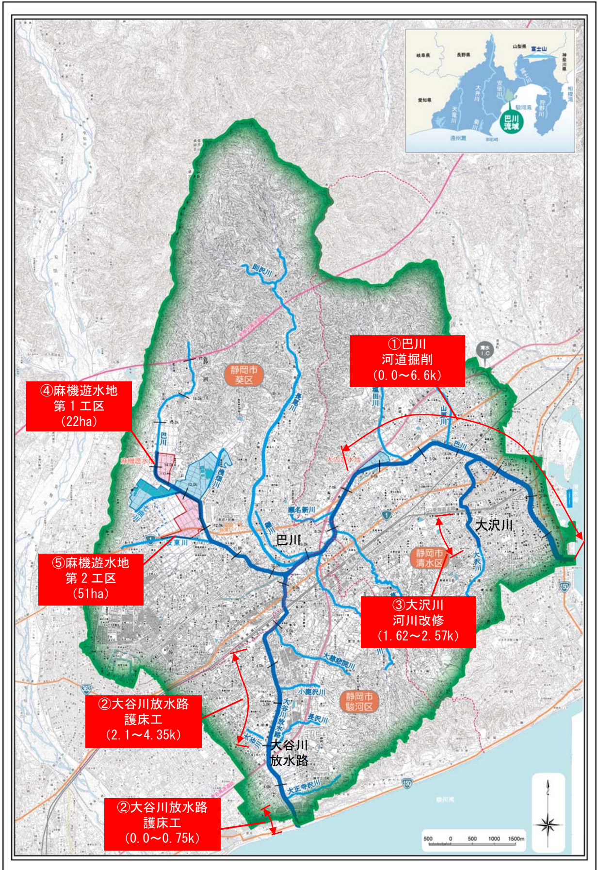
図 3.1 河川整備位置図
