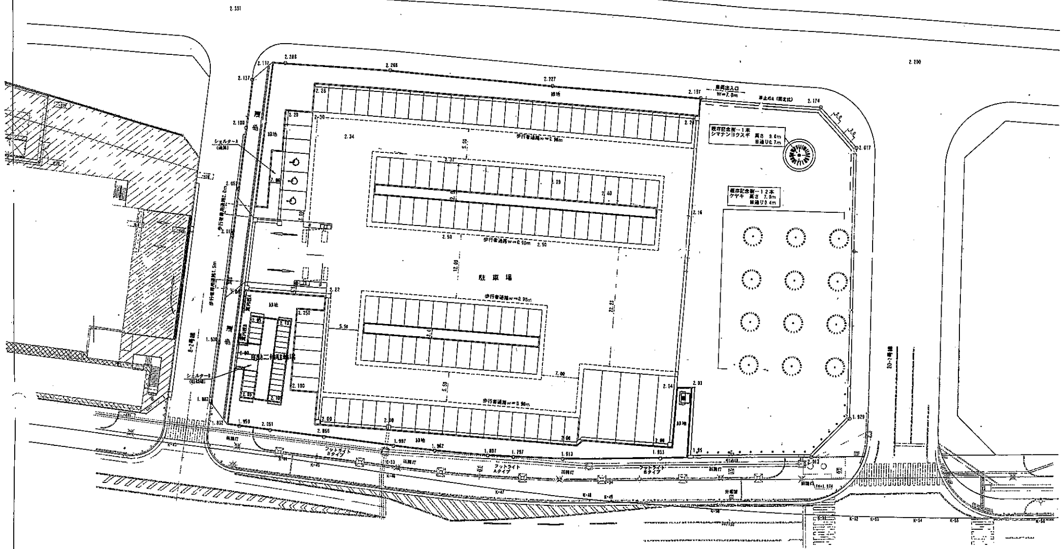
既存記念樹配置図 1 : 500
