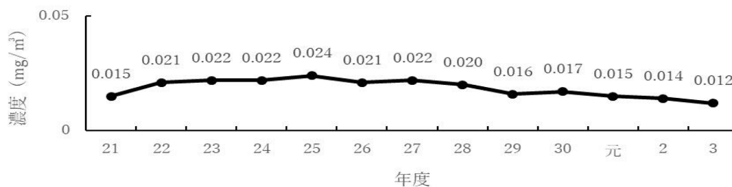
[図 3-14] 浮遊粒子状物質濃度年平均値の経年変化
