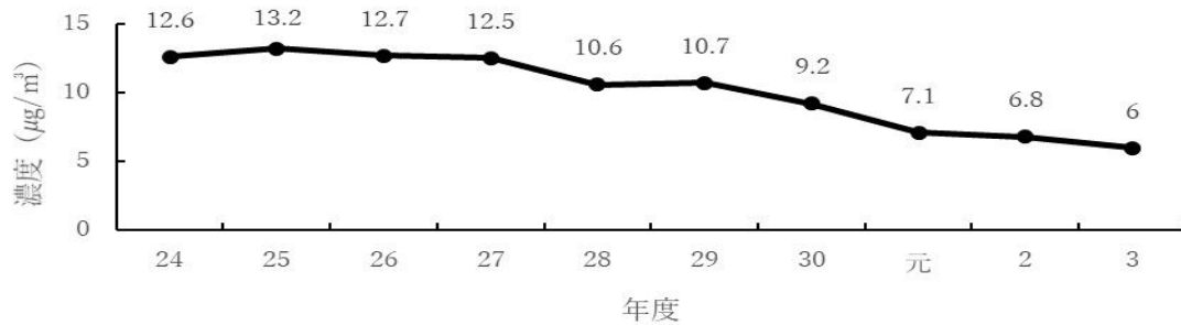
[図 3 - 15] 微小粒子状物質濃度年平均値の経年変化
