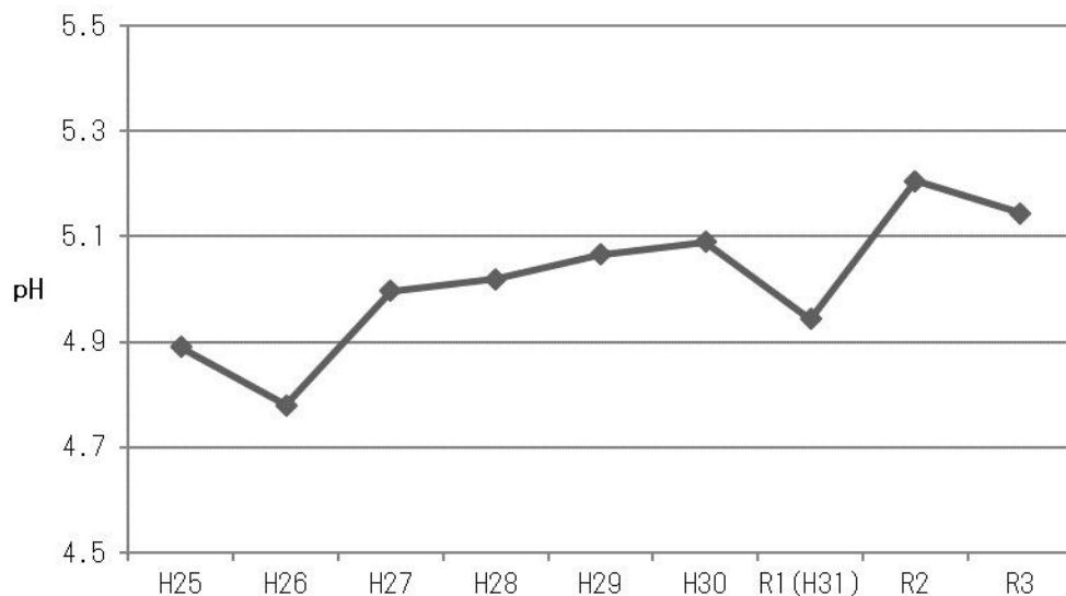
[図 3 - 21] pH の年平均値の推移 (平成 25 年度から令和 3 年度)
