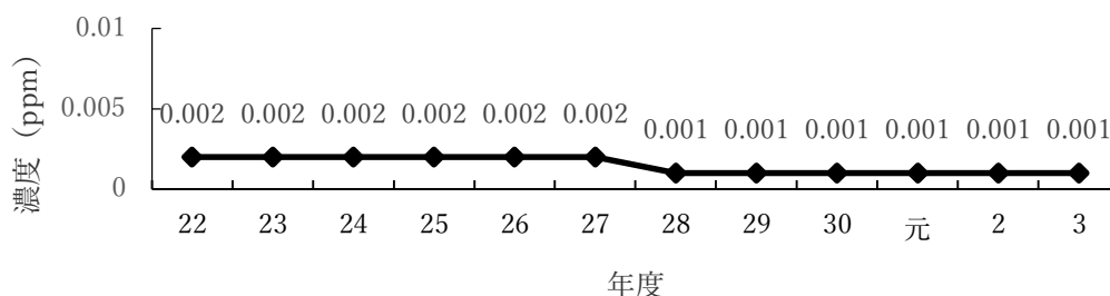
[図 3 - 4] 二酸化硫黄濃度年平均値の経年変化
