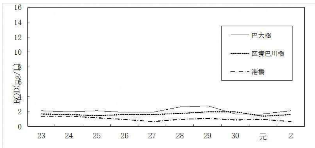
[図 3-25] 河川 BOD 環境基準 75% 水質値の推移 (その 3)
