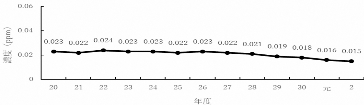
[図 3-13] 二酸化窒素濃度年平均値の経年変化
