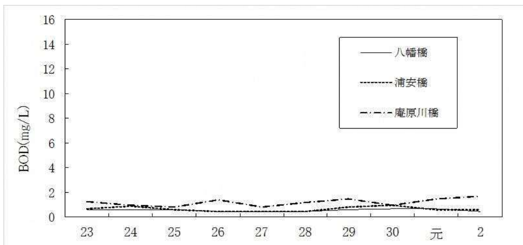
[図 3-26] 河川 BOD 環境基準 75% 水質値の推移 (その 4)
