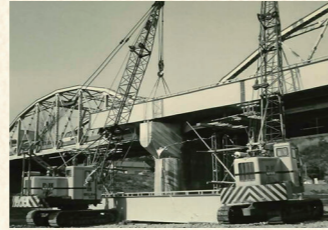
歩道橋設置工事 (写真提供:市川土木株)
