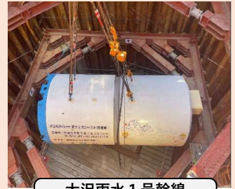
大沢雨水1号幹線 (シールドマシン)
