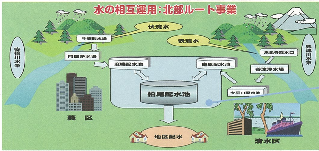
(仮称)中部配水池築造工事 平成25年度事業費 約8億円(総事業費約15億円) 災害等の緊急時に安倍川水系と興津川水系の水を相互に運用するため、(仮称)中部配水池を建設しました。平成26年4月に正式名称を「柏尾配水池」としました。
